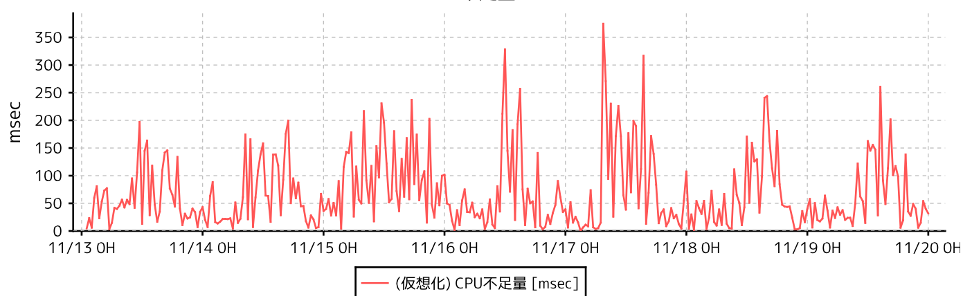
CPU不足量
