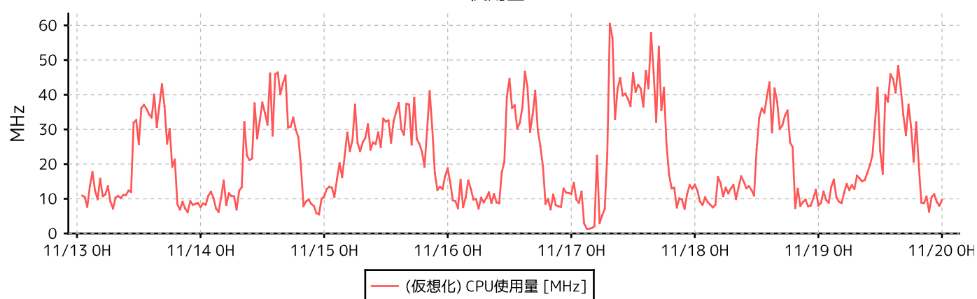
CPU使用量
