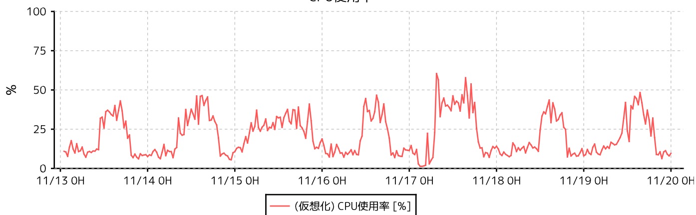
CPU使用率
