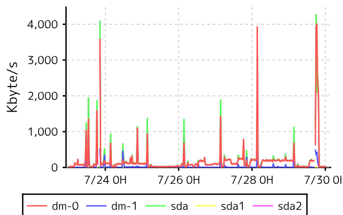
デバイス別ディスクI/O量
