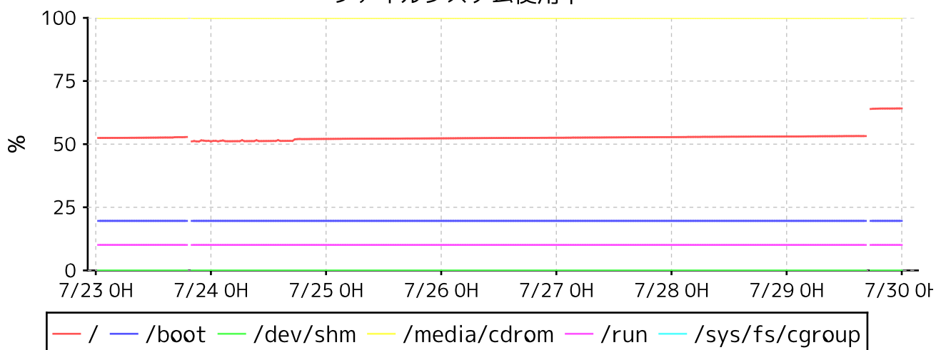
ファイルシステム使用率
