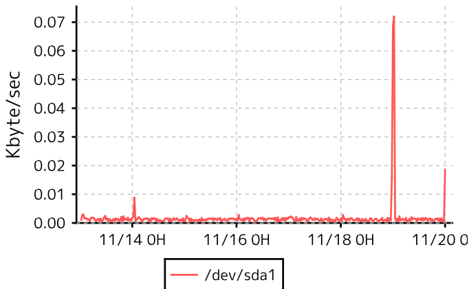
デバイス別ディスクI/O量(読み込み)
