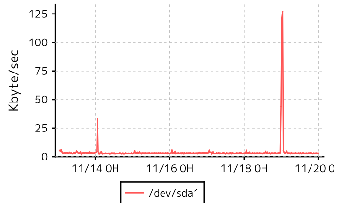
デバイス別ディスクI/O量(書き込み)
