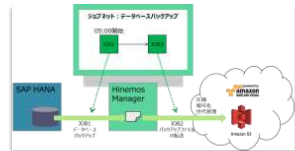
運用自動化テンプレートの例：クラウドへのバックアップ
