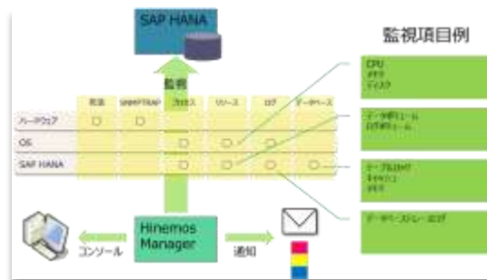
SAP HANA環境の監視概要
